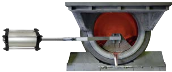
▲ Compuerta / Gate
